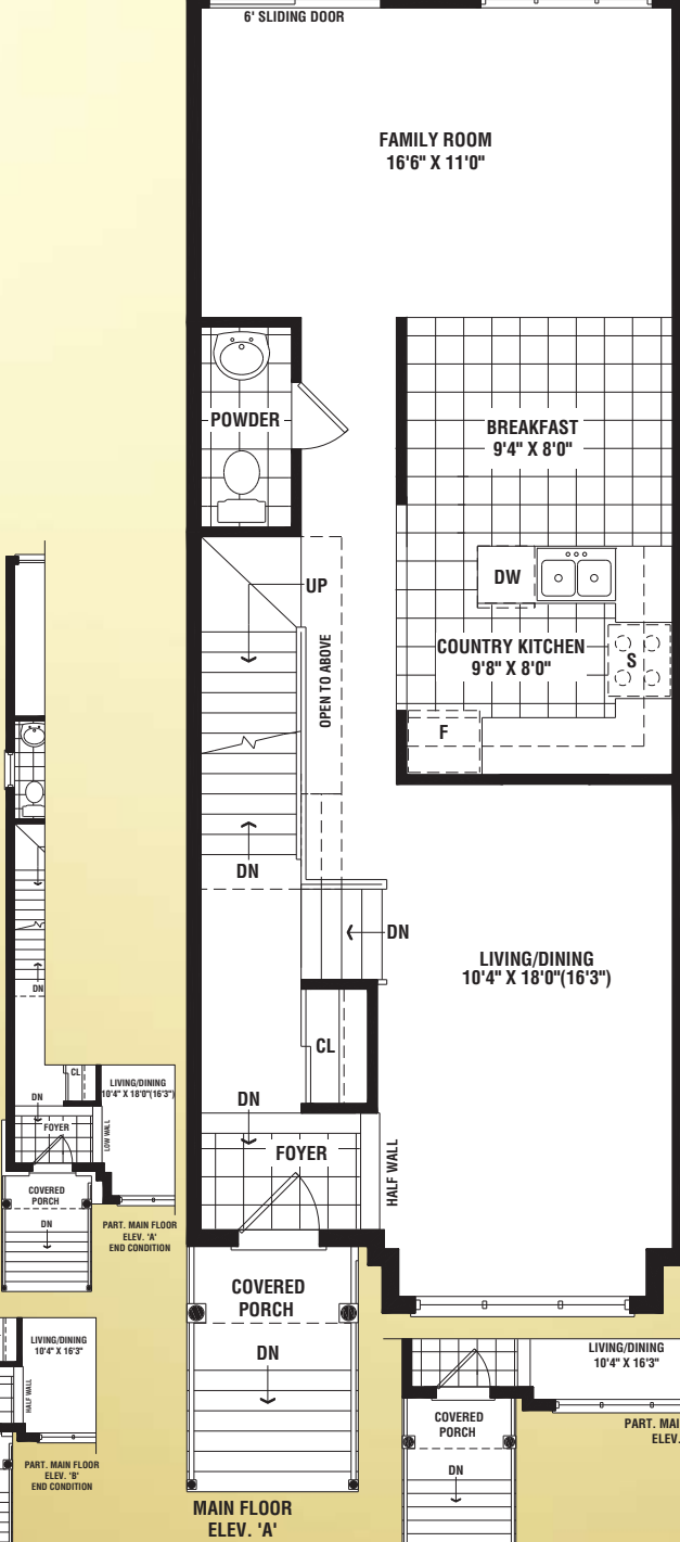
Elev. A
